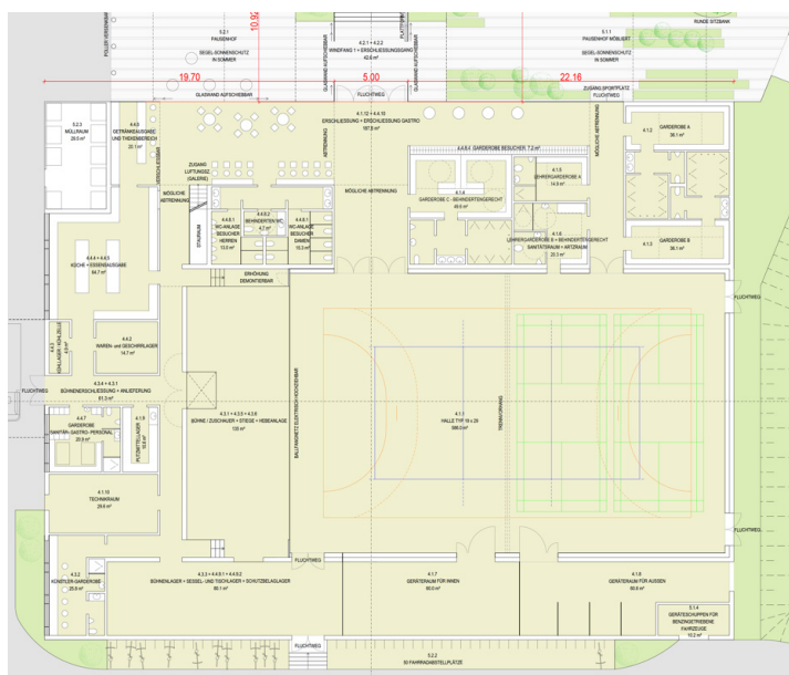
Grundriss von Architekt DI Erwin Kaltenegger
